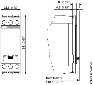
COV.11 透明密封盖
