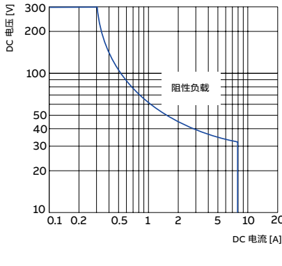
带2 c/o触点的型号
