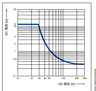
CR-M, 2 c/o触点
