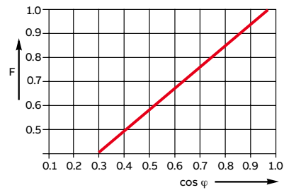
降容系数 - 感性交流负载下的F
