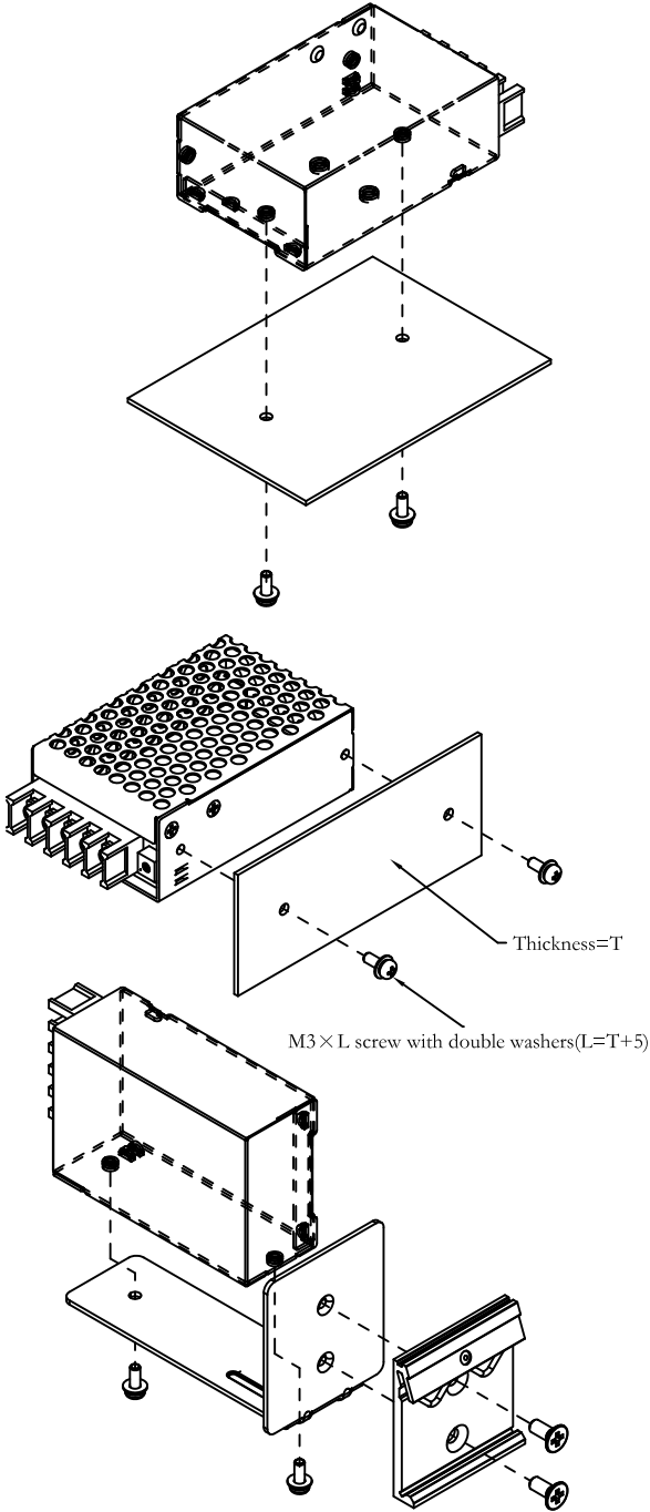
L型支架式导轨安装
