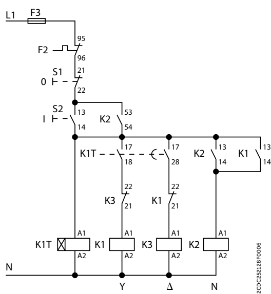
控制电路图
