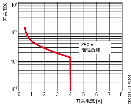
触点寿命
