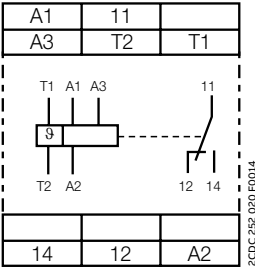
CM-MSS.13x
