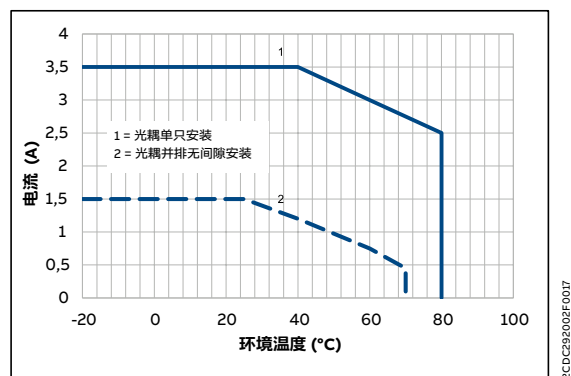
CR-P Triac输出
