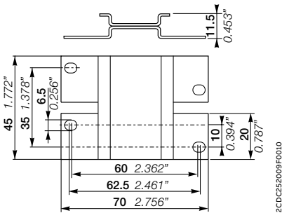
ADP.02 - 螺钉安装适配器
