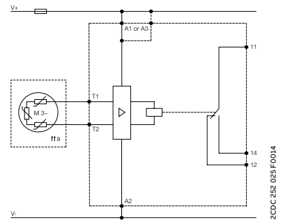
CM-MSS.13x
