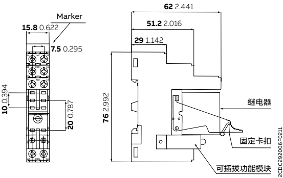
CR-PLS - 螺钉连接
