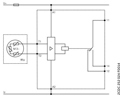
CM-MSS.12x
