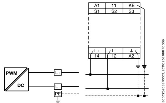
2线制直流系统
