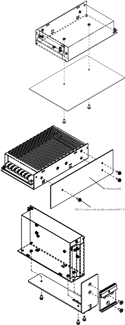
L型支架式导轨安装
