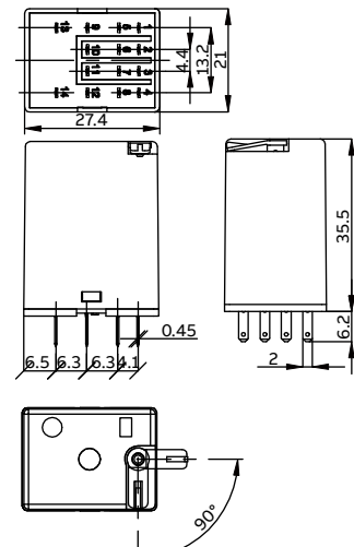
CR-M继电器, 4 c/o触点
