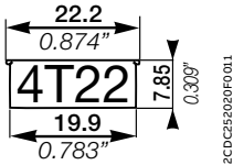
MAR.12 - 设备标识牌 (有DIP开关)
