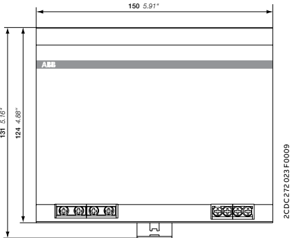
CP-T 24/20.0, CP-T 48/10.0
