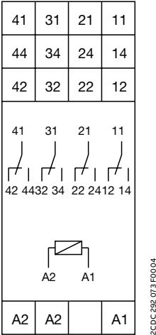
CR-M4LS, CR-M4LP
