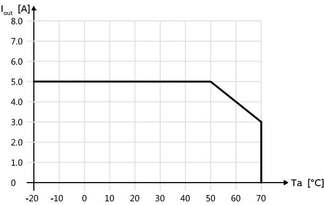
CP-PX 5/5.0
