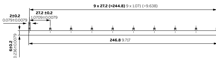
CR-MJ短接条
