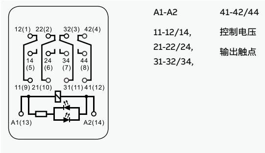
CR-MX, 4 c/o (SPDT) 触点, 带LED指示灯, 交流线圈
