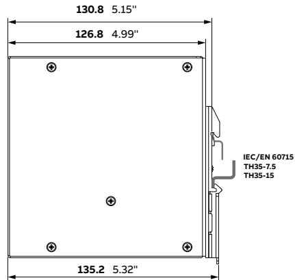
CP-S.1 24/3.0
