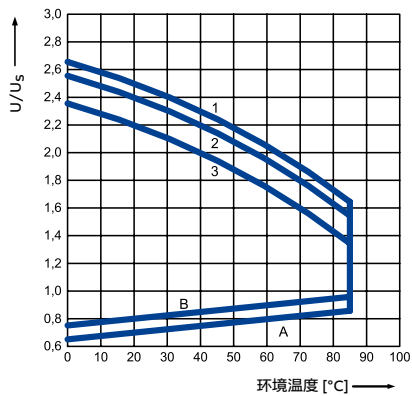
直流线圈的工作电压范围
