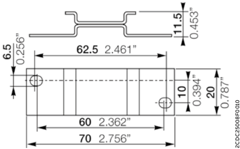
ADP.01 螺钉安装适配器
