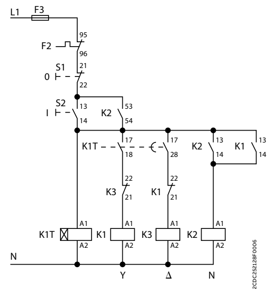
控制电路图
