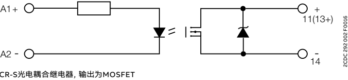
CR-S光电耦合继电器，输出为MOSFET
