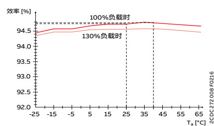
环境温度的典型效率
