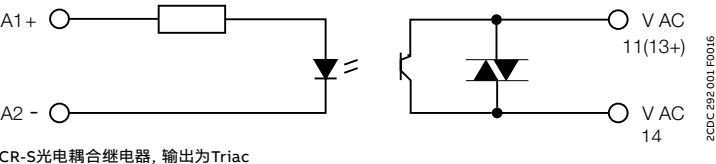
CR-S光电耦合继电器，输出为Triac
