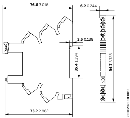
CR-S底座 - 弹簧连接
