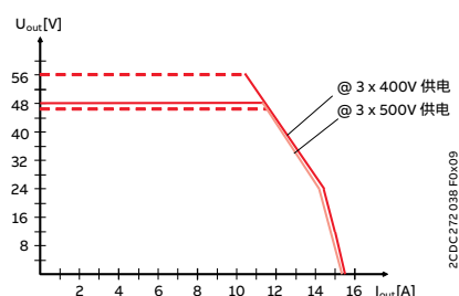
CP-T 48/10.0 U/I特性曲线
