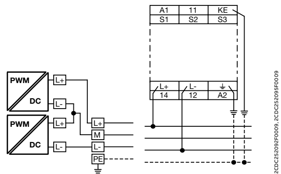
3线制直流系统
