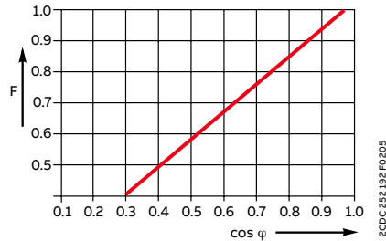
感性AC负载的降容系数F
