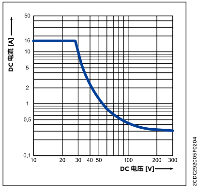
CR-P, 1 c/o触点
