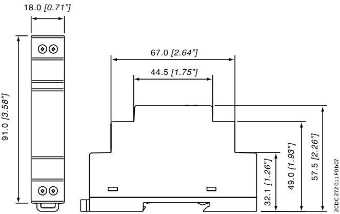
CP-D 12/0.83, CP-D 24/0.42
