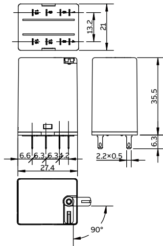
CR-M继电器, 2 c/o触点
