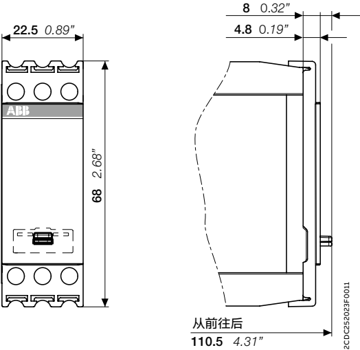
密封盖 COV:11
