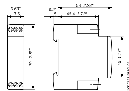
1 c/o或2 n/o触点输出的CT-D模块
