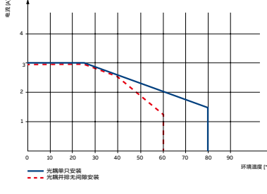
CR-S MOS-FET输出降容曲线
