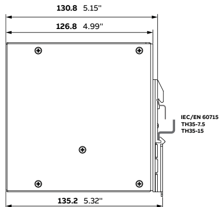
CP-S.1 24/10.0
