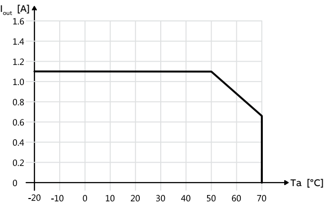
CP-PX 24/1.1
