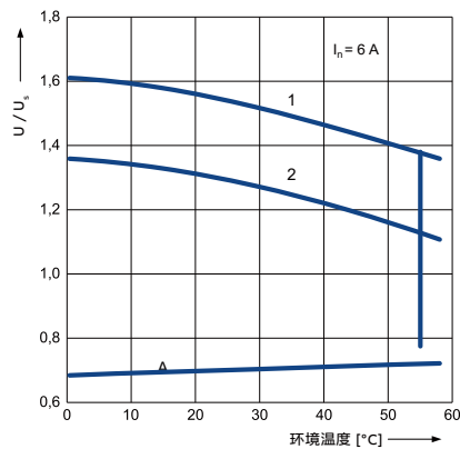
交流线圈的工作电压范围 - 4 c/o
