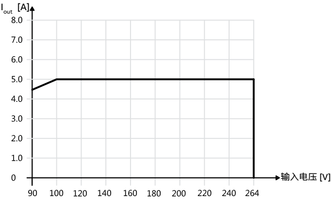
CP-PX 5/5.0
