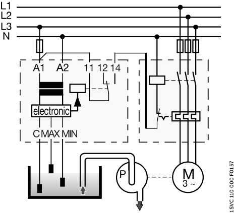
液位控制-抽干
