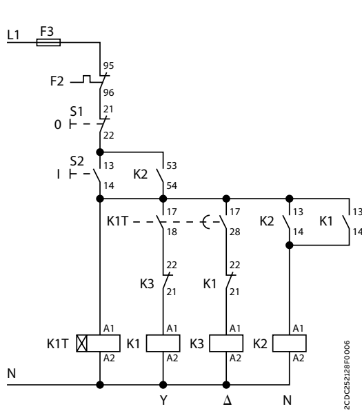
控制电路图
