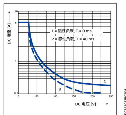
CR-M, 4 c/o触点
