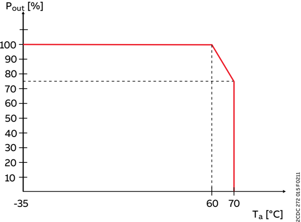
CP-E 12/10.0, CP-E 24/5.0
