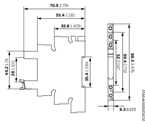
CR-S底座 - 螺钉连接
