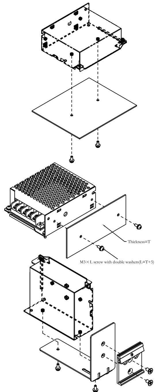
L型支架式导轨安装
