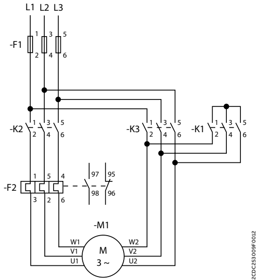
电源电路图
