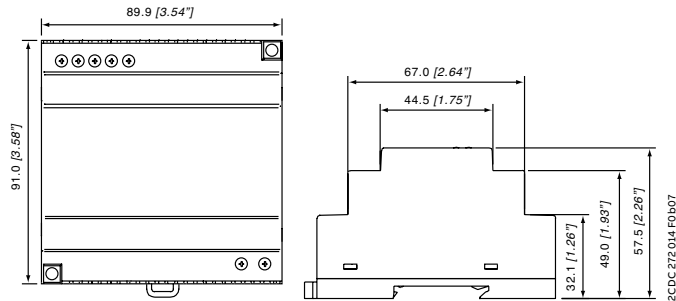
CP-D 24/4.2
