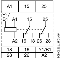
CT-MFD.21
