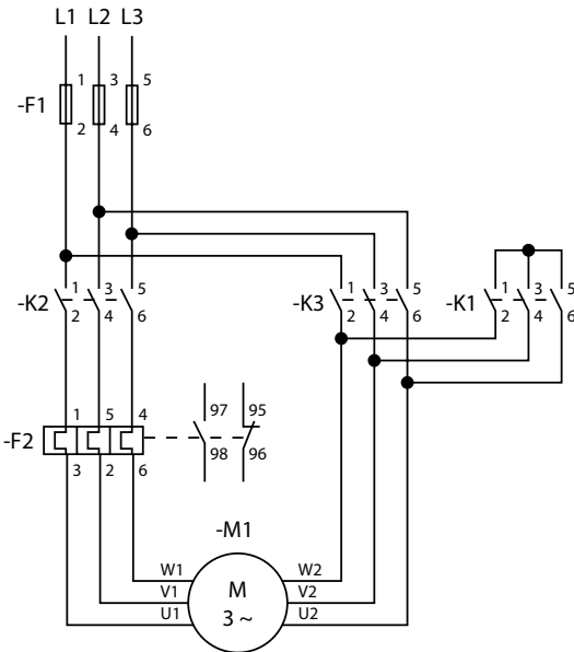
电源电路图
