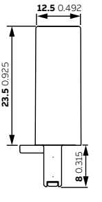
CR-P/Mxx功能模块
