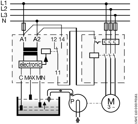
液位控制 - 加注 - 选择功能 "↑" (UP)
