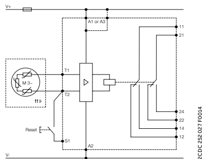
CM-MSS.23x
