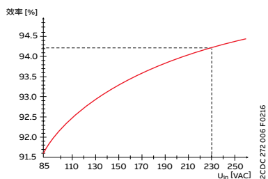
AC输入电压的典型效率
