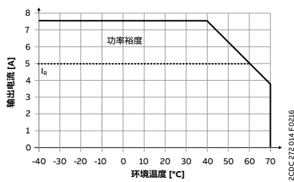
CP-C.124/5.0-C
