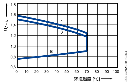
交流线圈的工作电压范围
