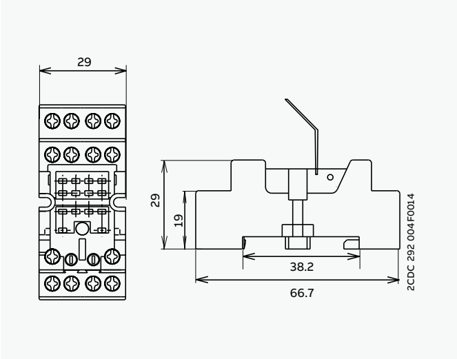
CR-MxSFB
