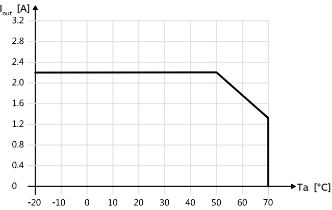
CP-PX 24/2.2
