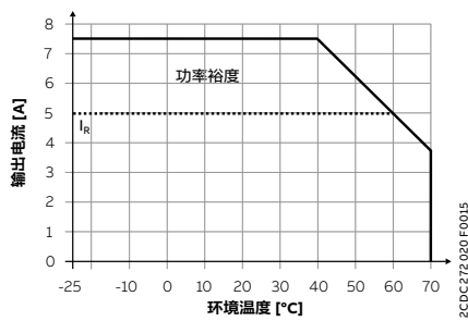
CP-C.124/5.0, CP-C.124/5.0-L
