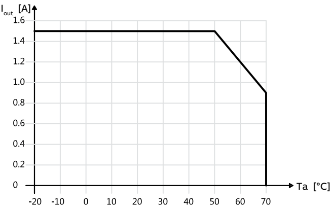
CP-PX 24/1.5
