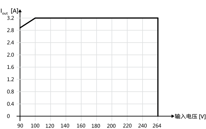
CP-PX 24/3.2
