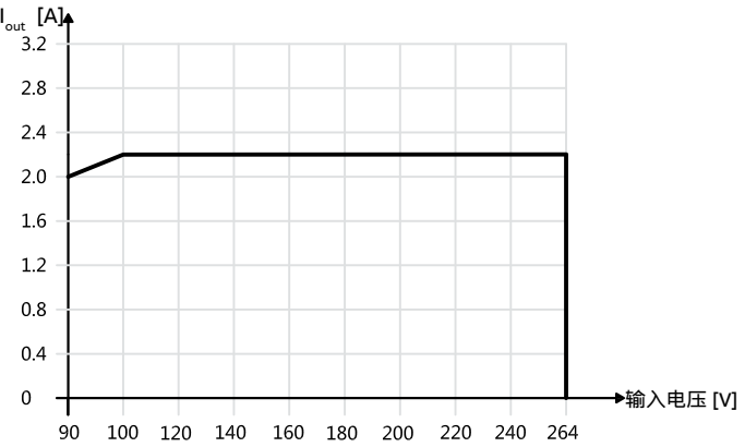
CP-PX 24/2.2
