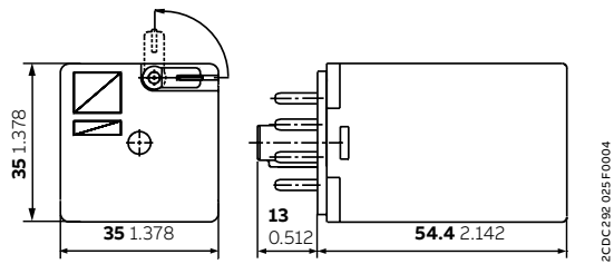
CR-U继电器, 2 c/o触点
