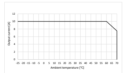
CP-S.1 24/10.0
