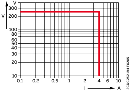
AC负载 (阻性)
