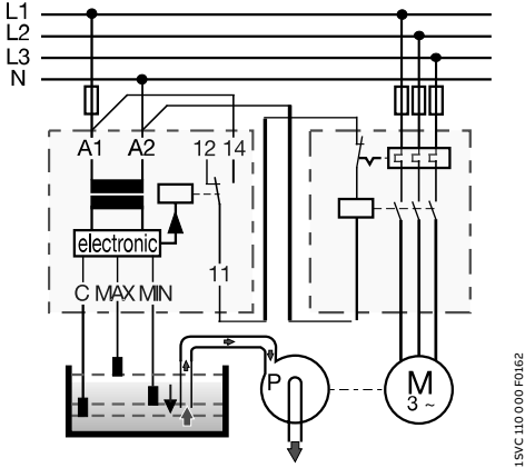
液位控制 - 抽干 - 选择功能 "↓" (Down)
