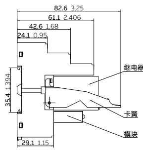
CR-M继电器, 3 c/o触点
