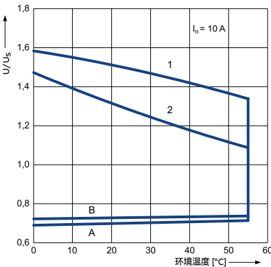
交流线圈的工作电压范围 - 3 c/o
