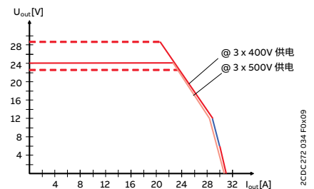
CP-T 24/20.0 U/I特性曲线
