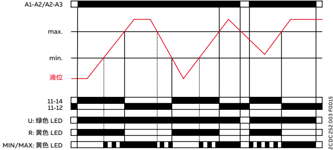
加注: CM-ENS.2x
