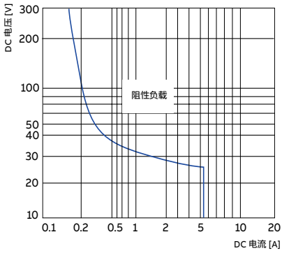
带1 n/o、1 n/c或1 c/o触点的型号
