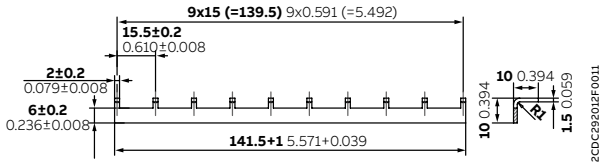
CR-PJ短接条
