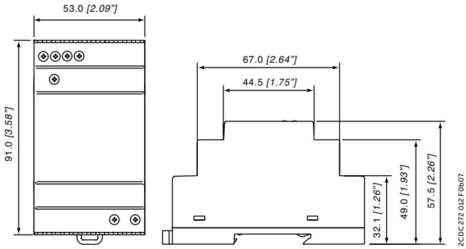
CP-D 12/2.1, CP-D 24/1.3
