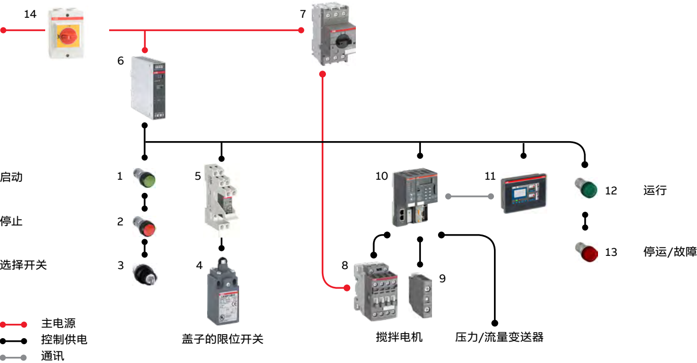
应用案例：搅拌机（电机功率 / 启动：3 kW/ 直接在线启动（DOL））
