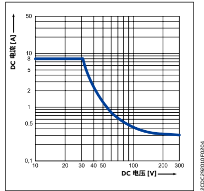
CR-P, 2 c/o触点
