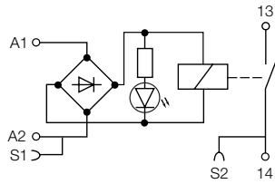
RB (R) 111-24VUC
