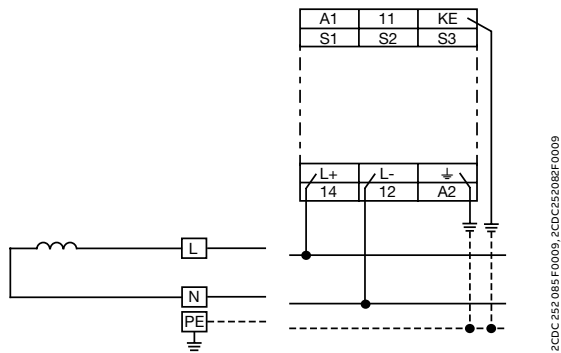
2线制交流系统
