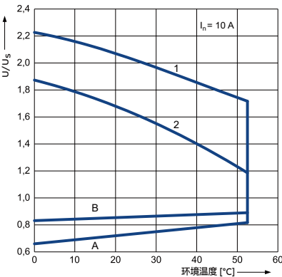
直流线圈的工作电压范围 - 3 c/o
