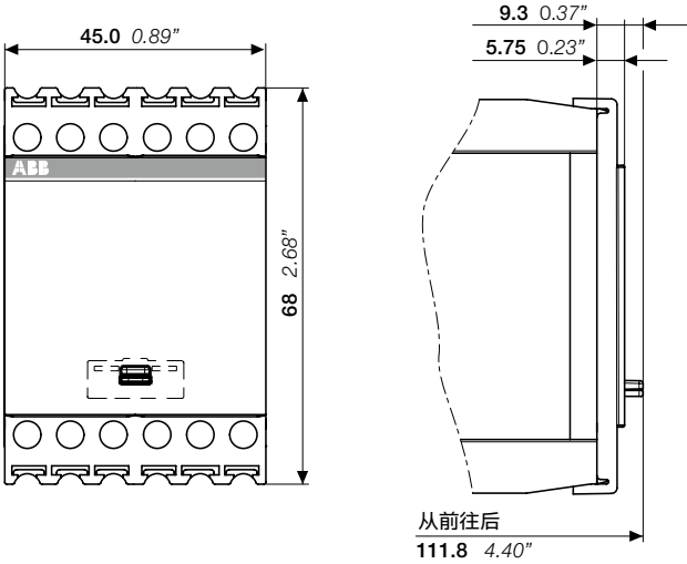
密封盖 COV: 12
