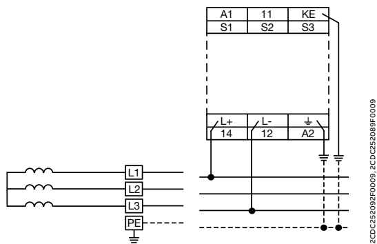
3线制交流系统
