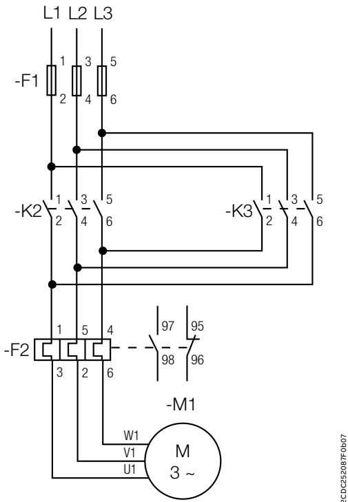
供电回路图
