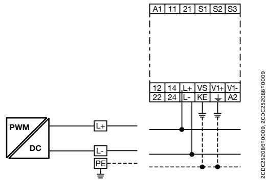
2线制直流系统
