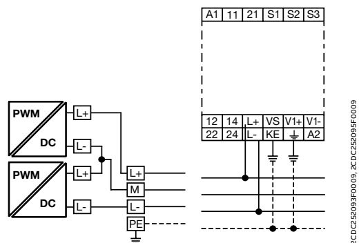
3线制直流系统
