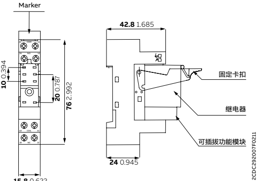
CR-PSS - 螺钉连接
