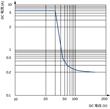
最大直流负载分断能力
