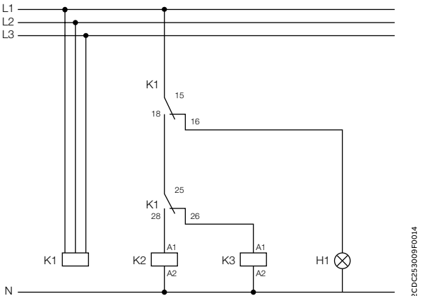
控制回路图 (K1 = CM-MPS.43或CM-MPN.xx)
