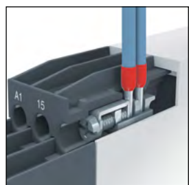
使用螺丝刀接线
