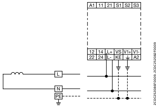
2线制交流系统
