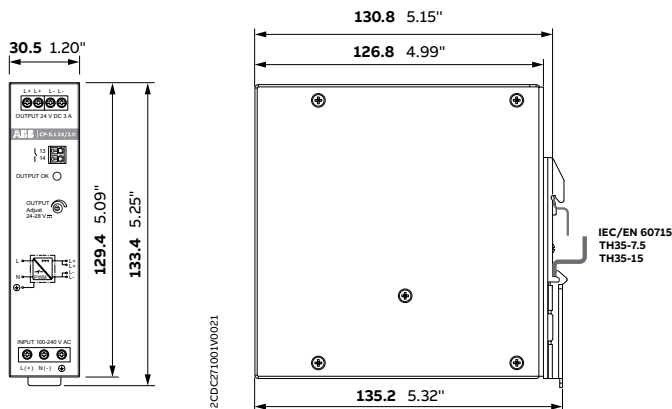
CP-S.1 24/5.0
