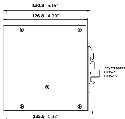
CP-S.1 24/40.0
