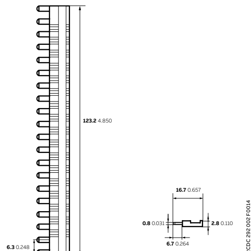
CR-SJB20-蓝色, CR-SJB20-红色, CR-SJB20-黑色短接条
