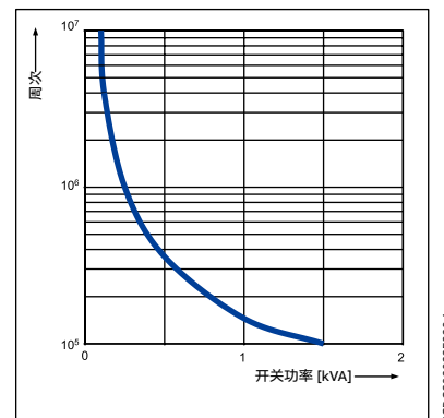
CR-M, 4 c/o触点
