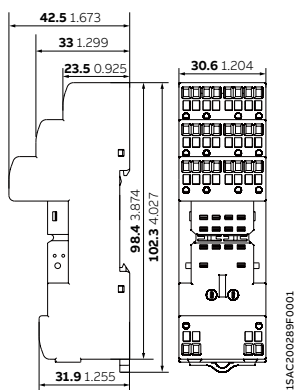
CR-MxLP - 弹簧连接
