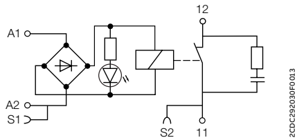
RB (R) 101R - 24VUC
