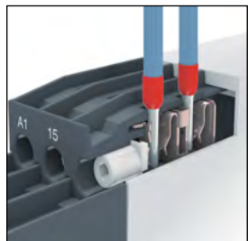
无需工具即可接线
