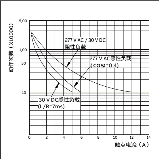
CR-CX, 1 c/o的型号
