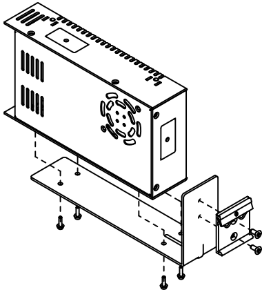
L型支架式导轨安装
