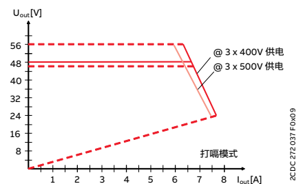
CP-T 48/5.0
