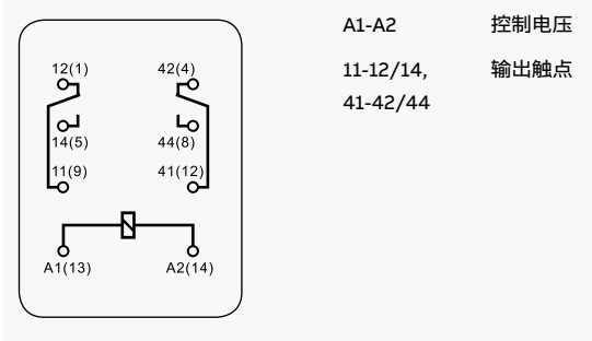
CR-MX, 2 c/o (SPDT) 触点, 不带LED指示灯, 交流线圈
