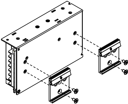
平板式导轨安装
