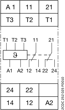
接线图
