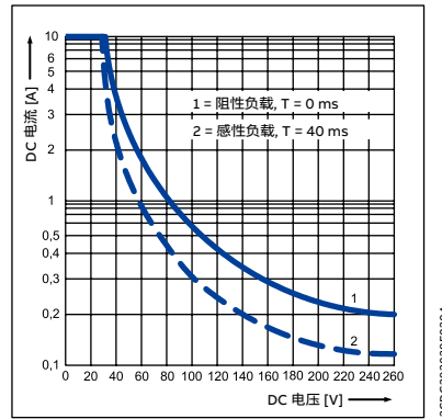
CR-U, 2和3 c/o触点
