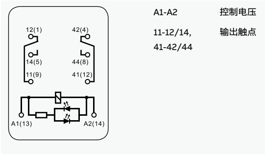
CR-MX, 2 c/o (SPDT) 触点, 带LED指示灯, 交流线圈
