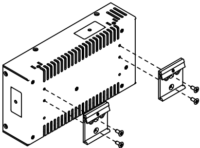
平板式导轨安装
