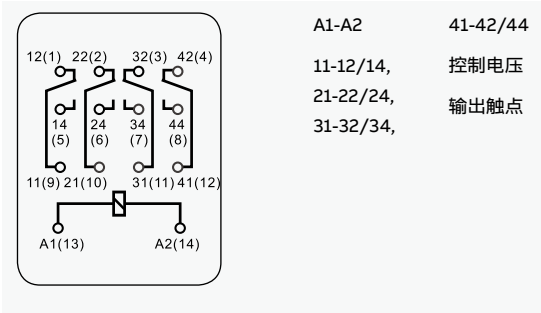
CR-MX, 4 c/o (SPDT) 触点, 不带LED指示灯, 交流线圈
