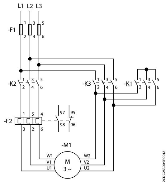
电源电路图
