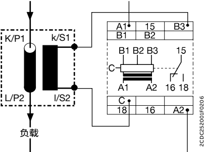
CM-CT
