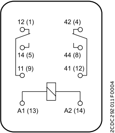
CR-M, 2 c/o触点
