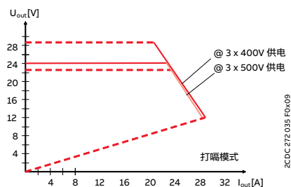
CP-T 24/20.0 打嗝模式
