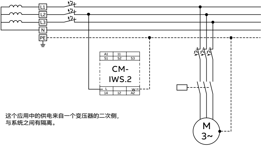
使用CM-IWS.2对四线IT交流系统进行接地故障/绝缘电阻监视
