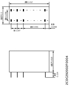
CR-P继电器
