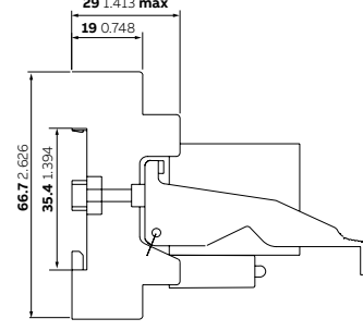
CR-M继电器, 4 c/o触点
