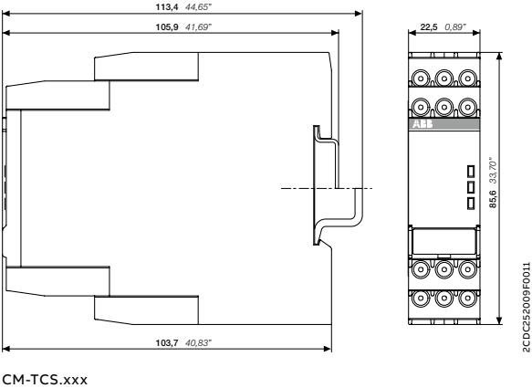
尺寸图 (mm和inch)
