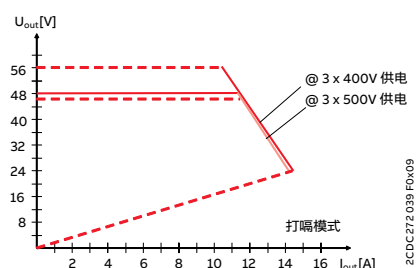
CP-T 48/10.0 打嗝模式
