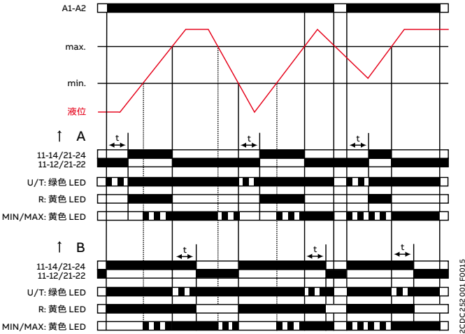
加注: CM-ENS.31
