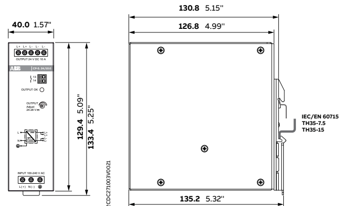
CP-S.1 24/20.0
