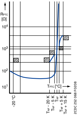
温度传感器特性
