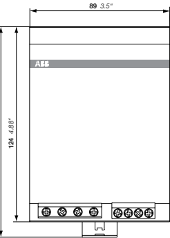
CP-T 24/10.0, CP-T 48/5.0
