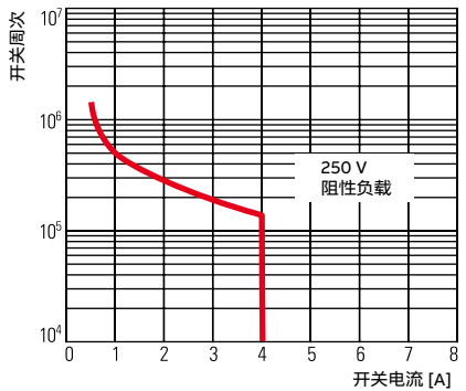
触点寿命
