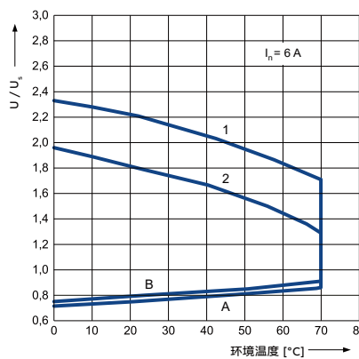
直流线圈的工作电压范围 - 4 c/o
