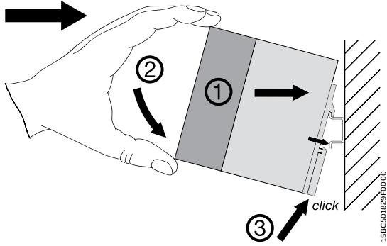
安装
