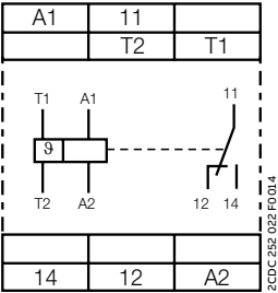
CM-MSS.12x
