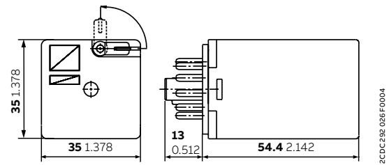
CR-U继电器, 3 c/o触点
