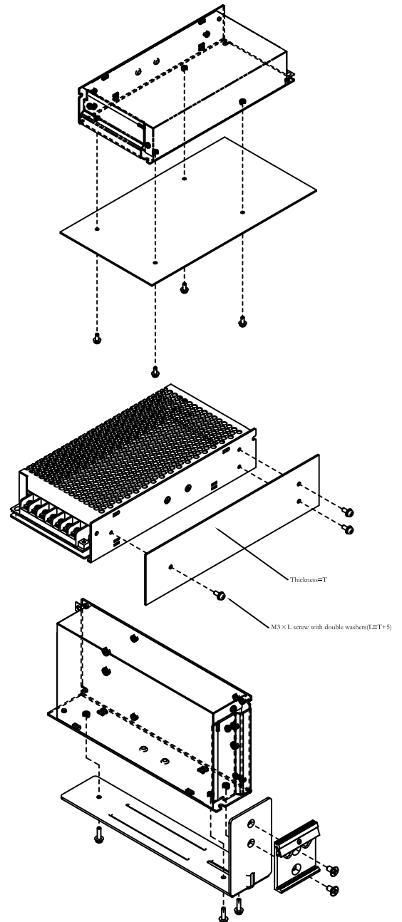
L型支架式导轨安装
