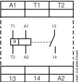
CM-MSE
