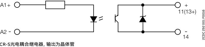
CR-S光电耦合继电器，输出为晶体管
