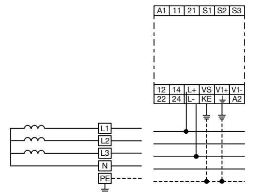
4线制交流系统
