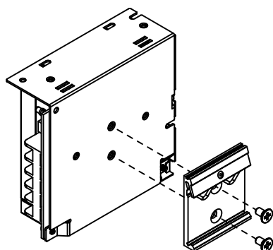
平板式导轨安装
