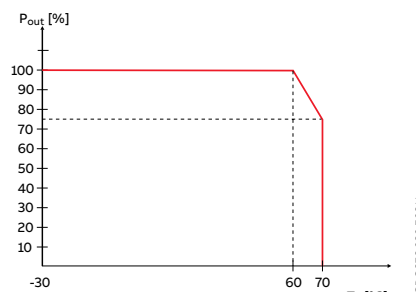
CP-T 24/20.0, CP-T 48/10.0
