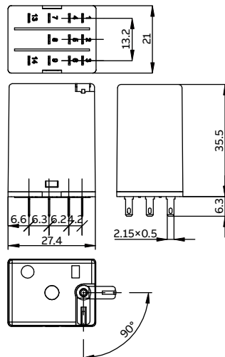
CR-M继电器, 3 c/o触点
