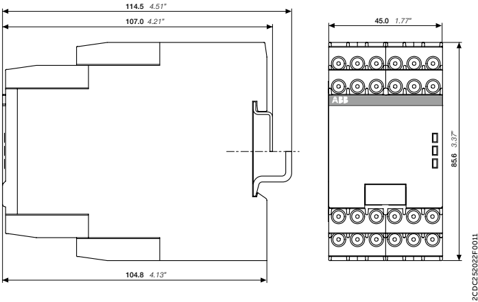
CM-IWN.x
