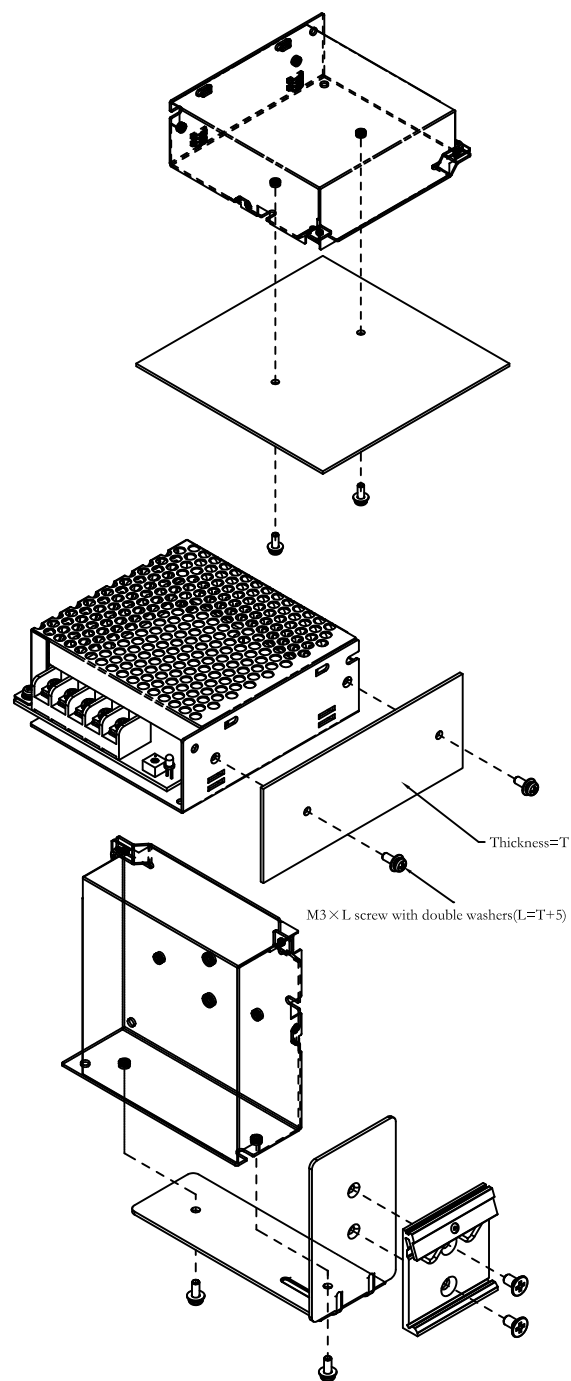
L型支架式导轨安装
