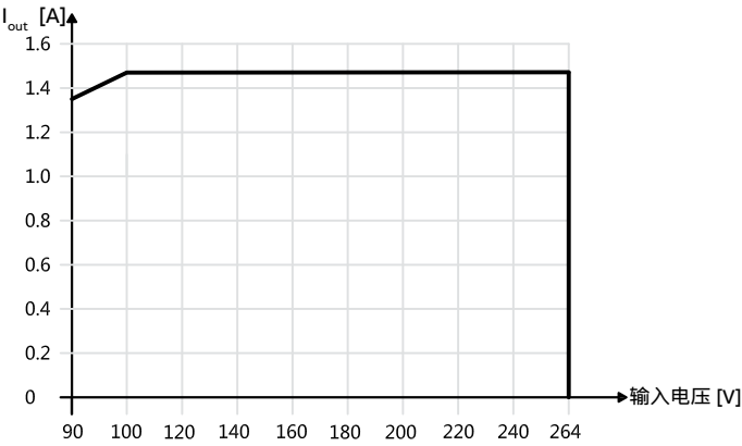
CP-PX 24/1.5
