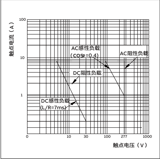
CR-CX, 2 c/o的型号
