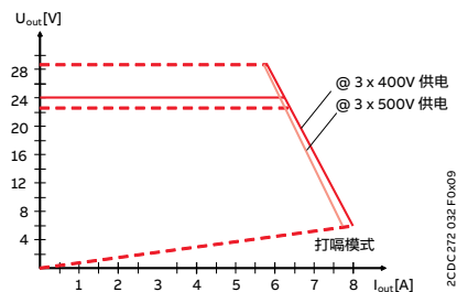
CP-T 24/5.0
