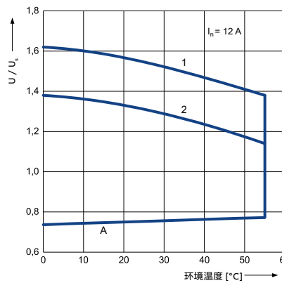
交流线圈的工作电压范围 - 2 c/o
