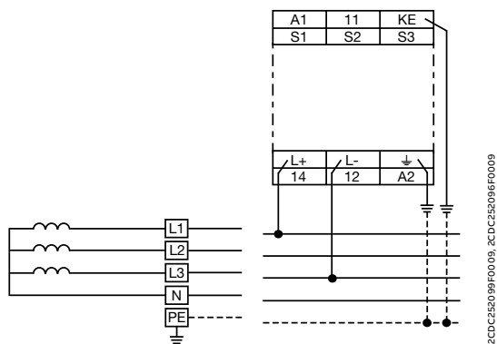
4线制交流系统
