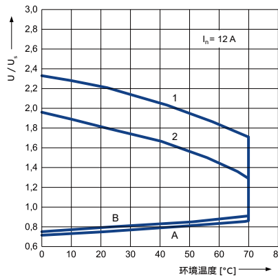
直流线圈的工作电压范围 - 2 c/o
