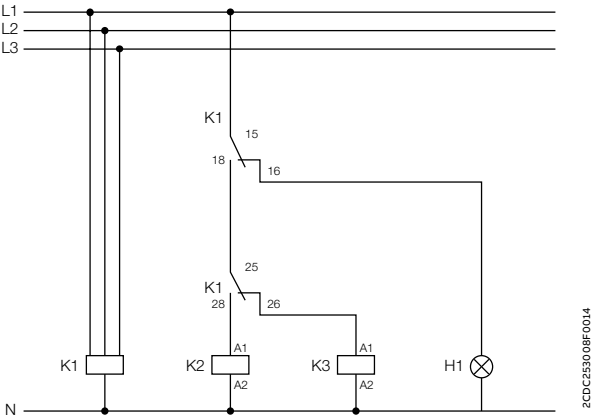
控制回路图 (K1 = CM-MPS.23)
