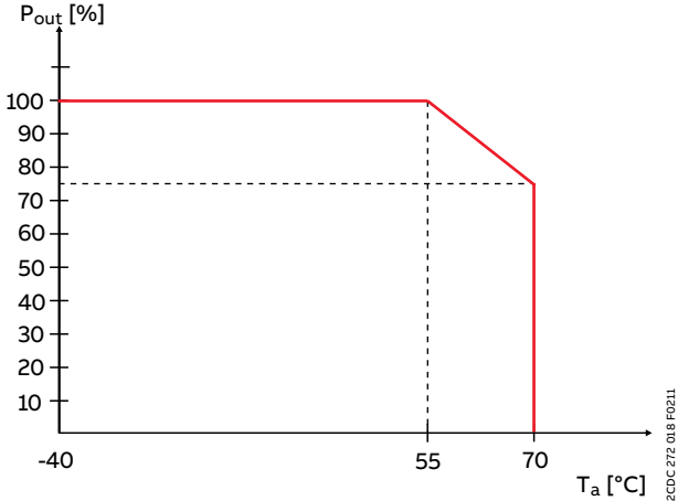
CP-E 24/20.0, CP-E 48/10.0
