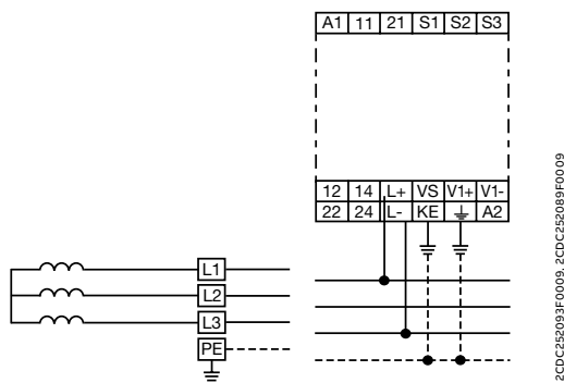
3线制交流系统
