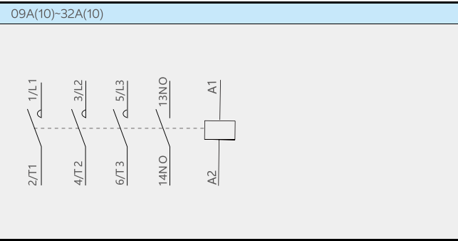
接线图
